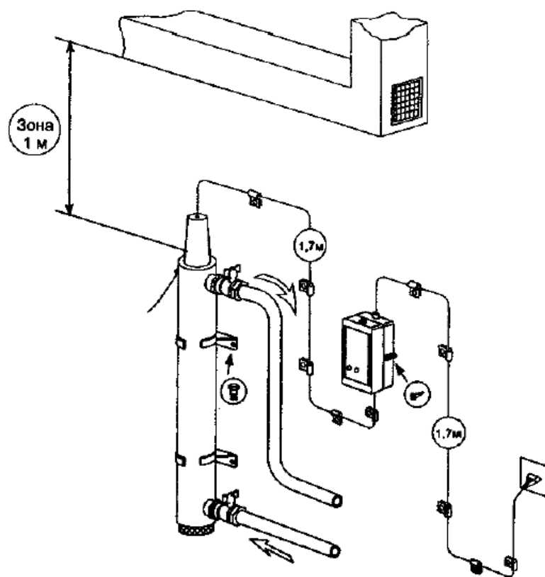
Пример монтажа установки в вертикальном положении
